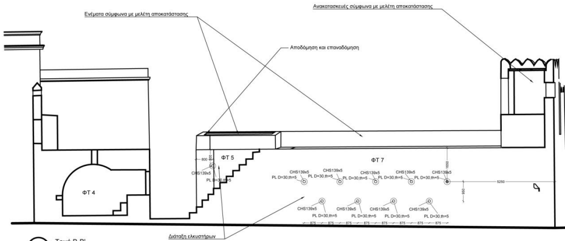
2 Τομή Β-Β' 1 : 100
