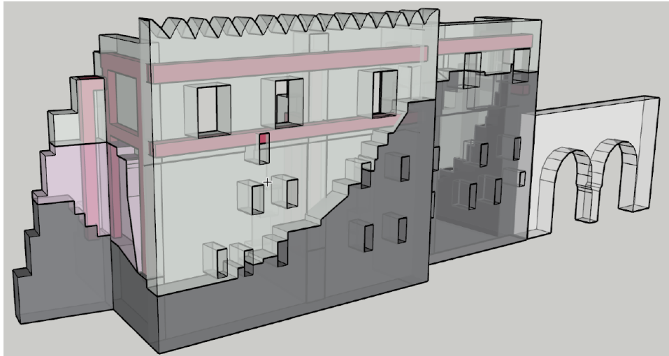
Εικ. 4: Πρόταση αποκατάστασης του τμήματος KM 1185 (μεγάλη οχύρωση). Με σκούρο γκρι παρουσιάζονται τα σωζόμενα τμήματα και με ανοικτό γκρι οι ανακατασκευές. Παράλληλα παρουσιάζονται με κόκκινο τα κατακόρυφα και οριζόντια διαζώματα από οπλισμένο σκυρόδεμα.
