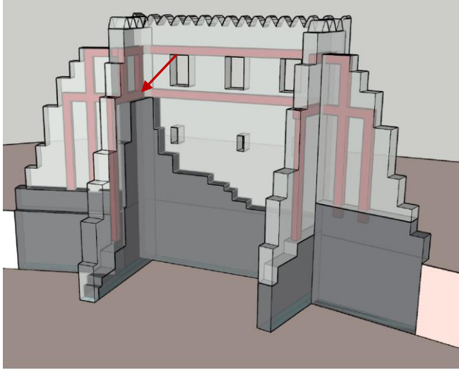
Εικ. 10: Πρόταση αποκατάστασης του τμήματος KM1179 (μικρή οχύρωση). Με σκούρο γκρι παρουσιάζονται τα σωζόμενα τμήματα και με ανοιχτό γκρι οι ανακατασκευές. Παράλληλα παρουσιάζονται με κόκκινο τα κατακόρυφα και οριζόντια διαζώματα από οπλισμένο σκυρόδεμα. Με κόκκινο βέλος επισημαίνεται η θέση όπου θα τοποθετηθούν βλήτρα που θα στερεώσουν περαιτέρω την ΝΑ γωνία της οχύρωσης με το υπερκείμενο οριζόντιο διάζωμα.
