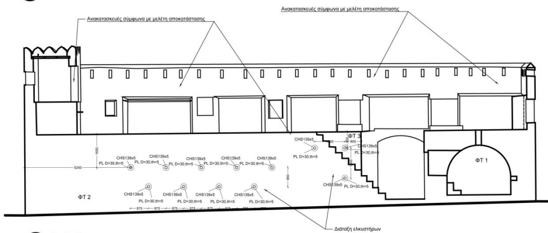
1 Τομή Α-Α' 1 : 100
