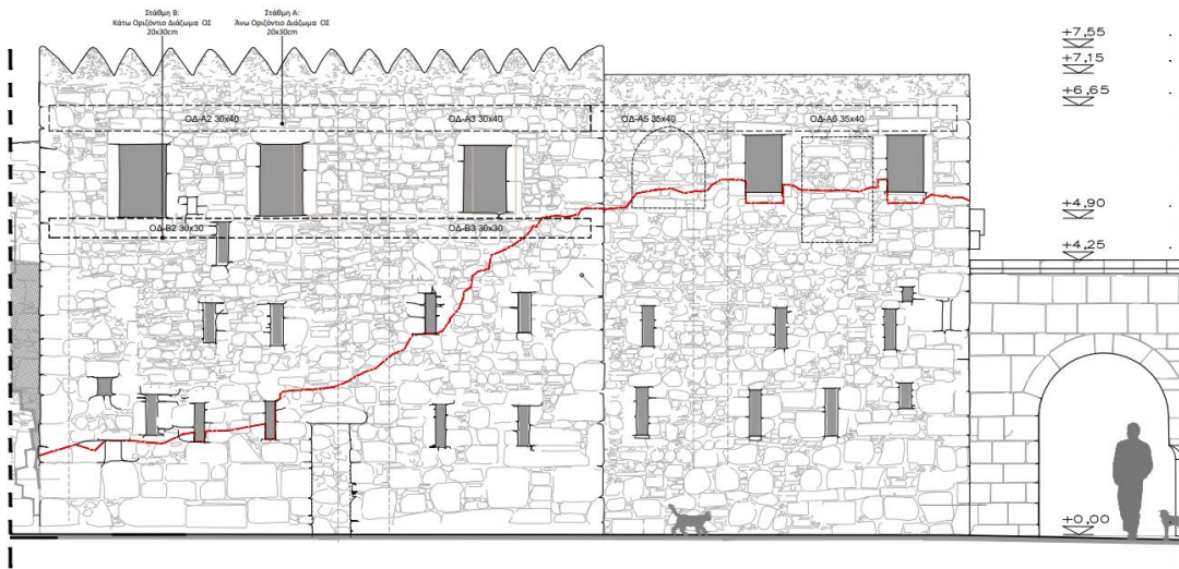
ΝΟΤΙΑ ΟΨΗ
