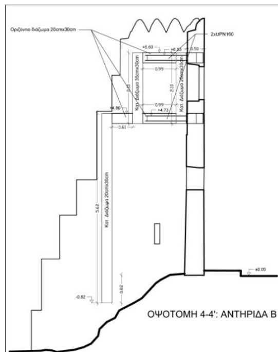
Εικ. 8: Σχεδιαστική απεικόνιση ανακατασκευών της τοιχοποιίας της κύριας όψης της μικρής οχύρωσης επί της οδού Ιπποκράτους (επάνω από την κόκκινη γραμμή) και κατασκευαστικές λεπτομέρειες αναδόμησης αντηρίδας της μικρής οχύρωσης.
