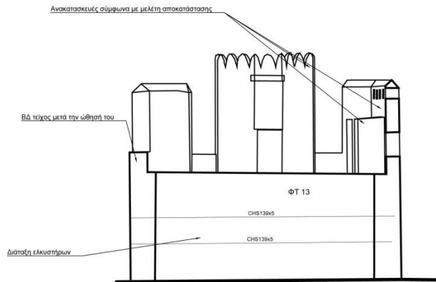
3 Τομή Γ-Γ 1 : 100
