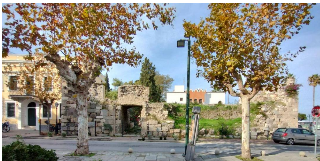
Εικ. 12: Η όψη του ΝΑ Προμαχώνα η οποία κατέρρευσε μετά το σεισμό του 2017.
