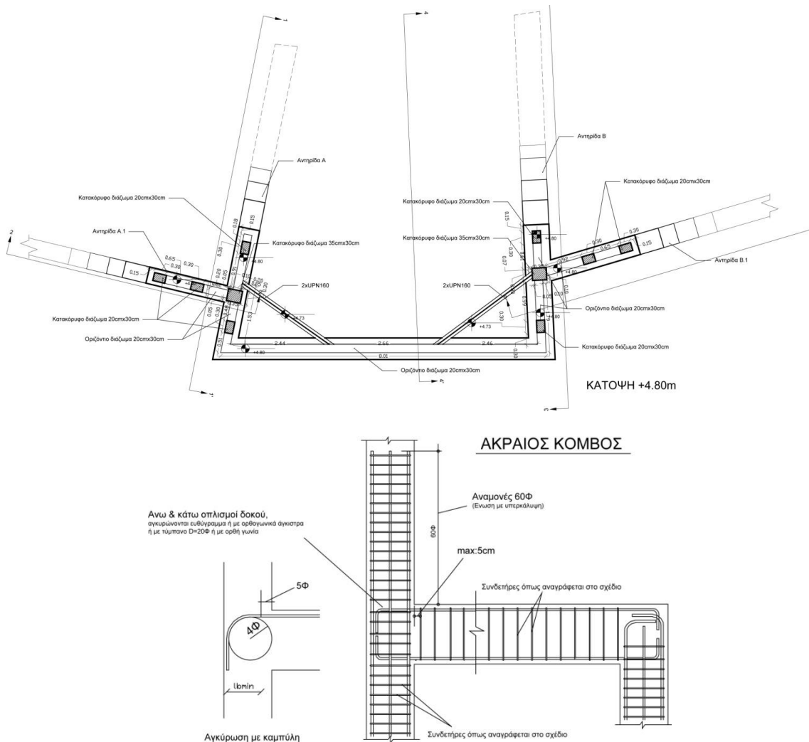
Εικ. 10: Κάτοψη μικρής οχύρωσης (επάνω) και λεπτομέρεια κόμβου αγκύρωσης οπλισμών διαζωμάτων (κάτω).
