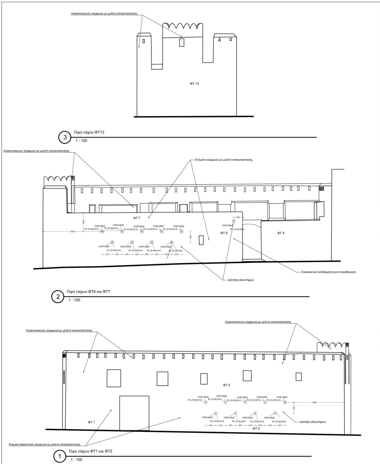
Εικ. 15: Σχεδιαστική απεικόνιση προτεινόμενων επεμβάσεων στον ΝΑ Προμαχώνα (όψεις).
