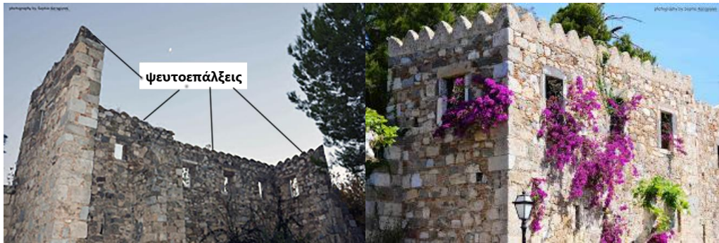
Εικ. 5: Ανακατασκευή ψευτοεπάλξεων στο τελείωμα των λιθοδομών των όψεων του τμήματος KM 1185 (μεγάλη οχύρωση), όπως φαίνεται σε εικόνες της οχύρωσης πριν την κατάρρευση.
