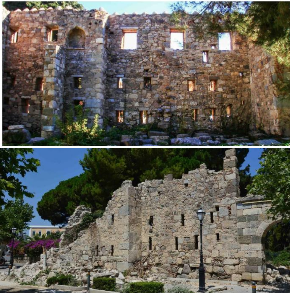
Εικ. 1: Τμήμα ΚΜ 1185 οχυρώσεων (μεγάλη οχύρωση) επί της οδού Ιπποκράτους πριν (επάνω, πίσω όψη) και μετά τον σεισμό του 2017 (κάτω, εμπρόσθια όψη).
