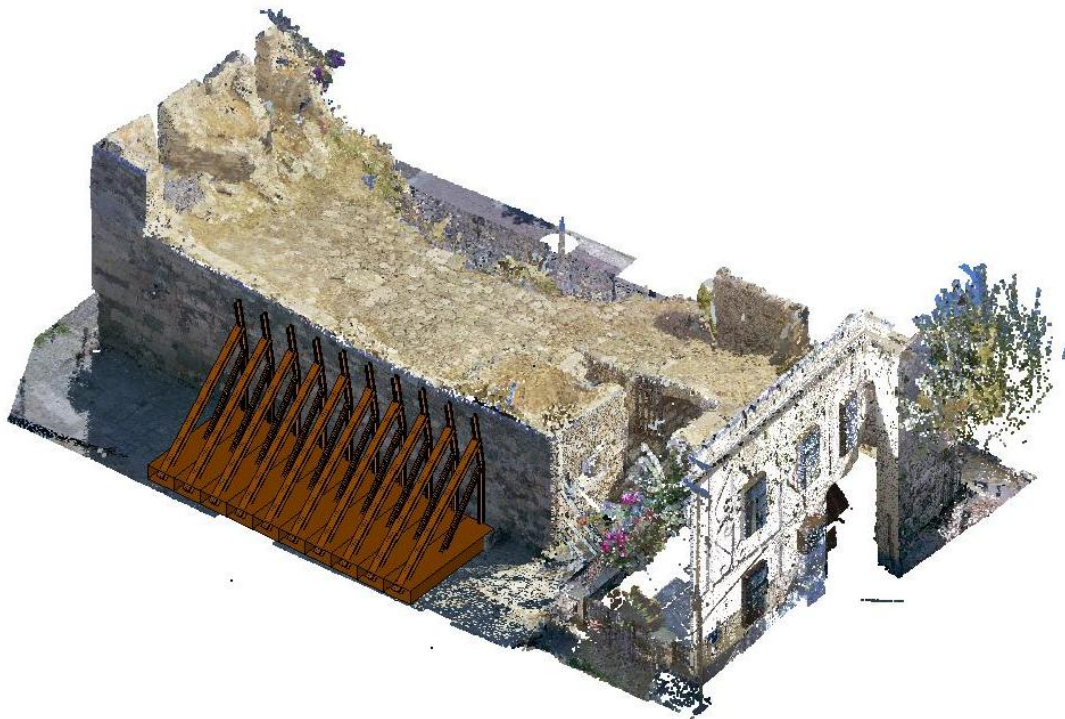
Εικ. 13: ΒΔ όψη του Προμαχώνα όπου το τείχος αποκλίνει από την κατακόρυφο και θα αναταχθεί με μηχανισμό ώθησης. Στη βάση της κάθε δοκού HEA240 του μηχανισμού τοποθετείται υδραυλικός γρύλος χειρός, δυνατότητας 20t σε βάρος και κατ' ελάχιστο 400mm διαδρομής εμβόλου. Οι γρύλοι αυτοί είναι πολύ συνηθισμένοι σε συνεργεία αυτοκινήτων και βαρέων οχημάτων και προσφέρουν τη δυνατότητα κλειδώματος σε συγκεκριμένη θέση. Η βάση του γρύλου συνδέεται με τη θεμελίωση πάλι με μεταλλικό πίστο. Ως εκ τούτου, δημιουργείται ένα ευσταθές τριαρθρωτό τόξο, το οποίο παράλληλα έχει δυνατότητα να μεταβάλλει τη γεωμετρία του ώστε να προσαρμοστεί στην επέκταση του εμβόλου και στην αλλαγή της θέσης του τείχους.
