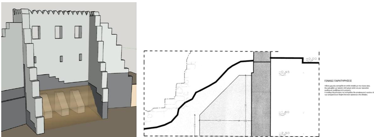
Εικ. 7: Πρόταση αποκατάστασης του τμήματος KM1179 (μικρή οχύρωση). Με σκούρο γκρι παρουσιάζονται τα σωζόμενα τμήματα και με ανοικτό γκρι οι ανακατασκευές. Παράλληλα φαίνονται και οι τρεις λίθινες αντηρίδες στη βάση της τοιχοποιίας οι οποίες θα καλυφθούν με χώμα (αριστερά). Κατασκευαστική λεπτομέρεια λίθινης αντηρίδας βάσης (δεξιά).
